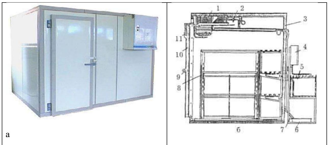
Рисунок 1.1 - Середньотемпературна камера КХС-2-6М
