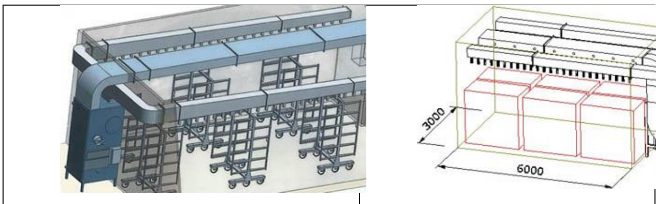
Рисунок 1.10 - Дефростаційно – морозильна камера з вертикальною подачею потоку повітря.
