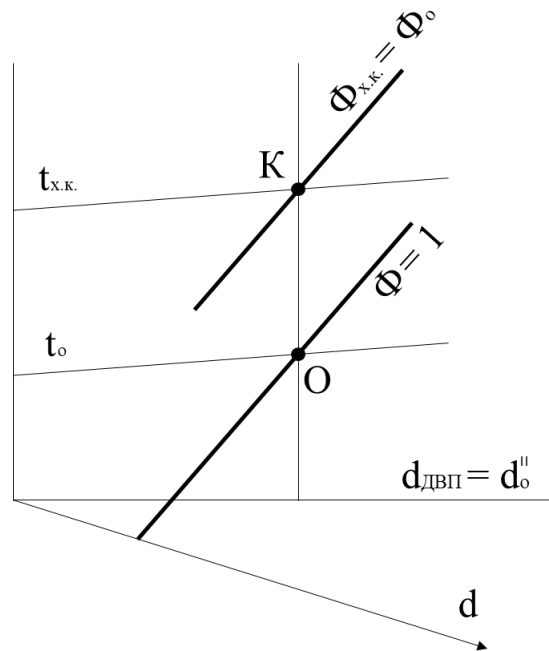
Рисунок 2.3 Рівнозважена вологість повітря в холодильній камері при відсутності виділення вологи
