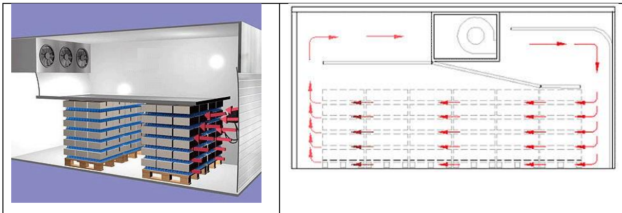
Рисунок 2.1 - Дефростаційно – морозильна камера з горизонтальною подачею потоку повітря .
