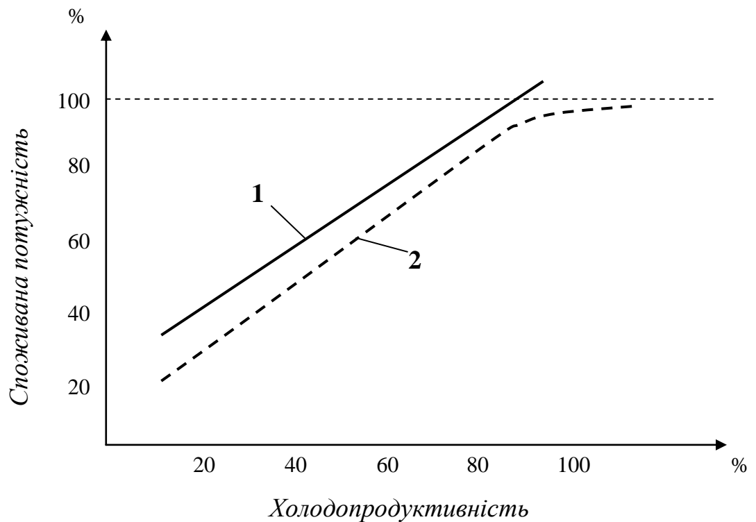
Рисунок 3.2 – Залежність споживаної потужності електроприводу від холодопродуктивності ХМ: 1 – контроль потужності за допомогою повзуна; 2 – контроль потужності за допомогою ТПЧ-АД
