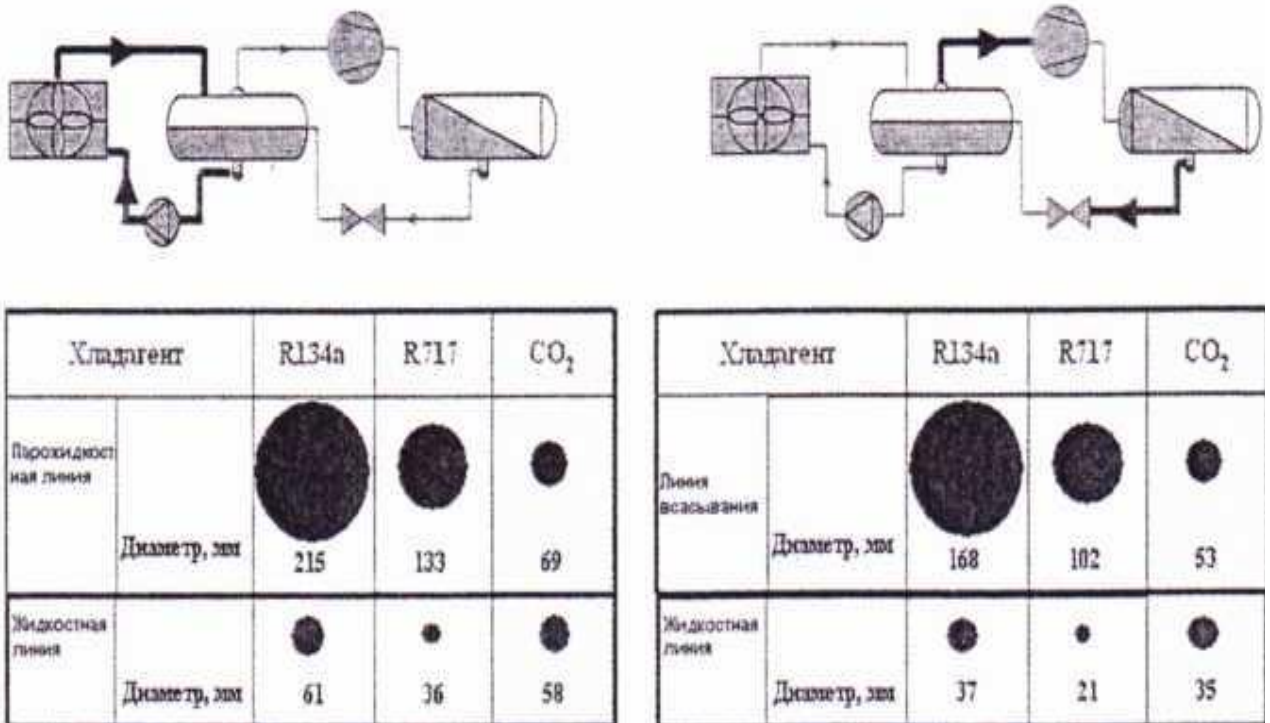
Рисунок 3.1 - Переваги застосування CO 2 з точки зору енергоефективності холодозабезпечення обладнання супермаркетингів
