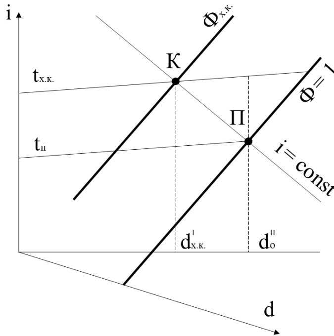
Рисунок 2.2 Стан вологого повітря в холодильній камері.
