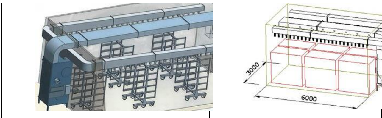
Рисунок 2.2 - Дефростаційно – морозильна камера з вертикальною подачею потоку повітря.
