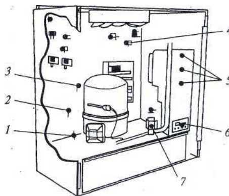
Рисунок 3.5– Локальні системи автоматика компресорних агрегатів: 1 - фільтр-осушувач; 2 - індикатор вологості; 3 - регулятор тиску усмоктування; 4 - регулятор тиску конденсації; 5 - регулятор швидкості обертання вентилятора, що обдуває конденсатор; 6- панель керування; 7- соленоїдний вентиль відтавання
