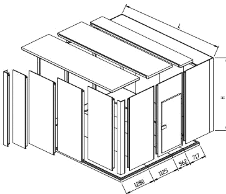
Рисунок 1.2 – Збірна холодильна камера
