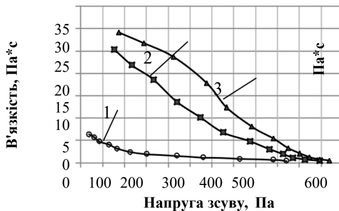
Рисунок 1 - Криві ефективної в'язкості модельних систем тіста з крохмалю після замішування: 1 – з камеддю гуару; 2 – з камеддю ксантану; 3 – з сумішшю камедей
